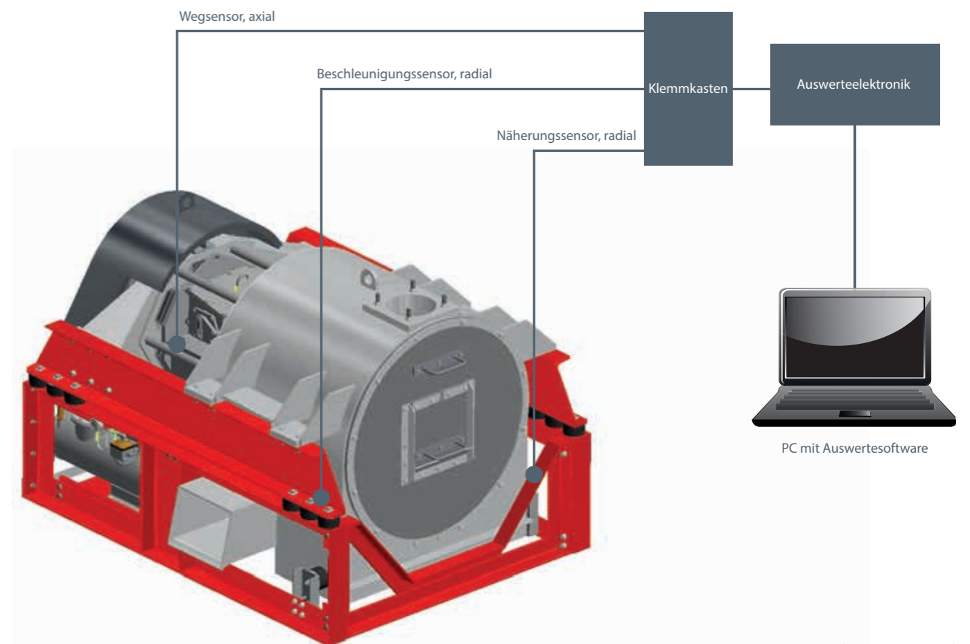
Schwingungs- und Auslenkungsmessung an HSG Zentrifugen
