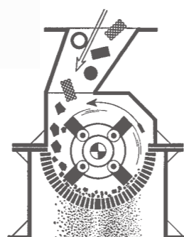
Princípio de trabalho do moinho de martelos
