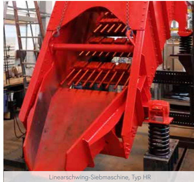
Linearschwing-Siebmaschine, Typ HR
